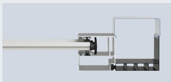
Rolovací vrata SB / TGT s profilem Decotherm S a plastovým větrným hákem
