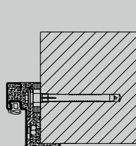
Rohová zárubeň se skrytou montáží pomocí hmoždinek
