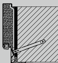
Obvodová zárubeň Diagonální upevnění do MW 175
