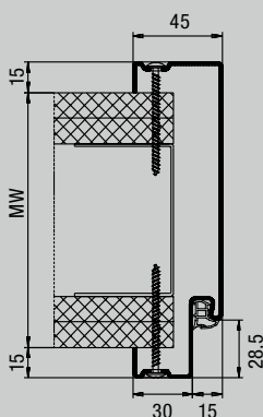
Profil 21120 Upevnění zrcadlovými šrouby
