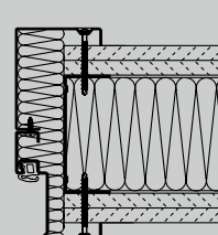
Rohová a přídavná zárubeň Montáž pomocí šroubů
