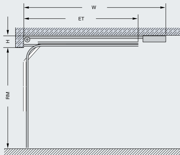
Sekční vrata s kováním L
